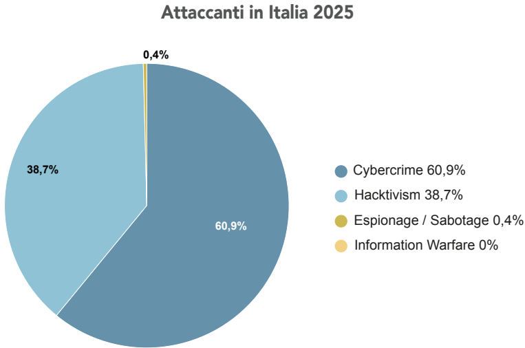
Fig. 27 - Attaccanti in Italia nel 2025
